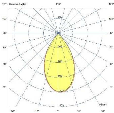
Светлоразпределителна диаграма
