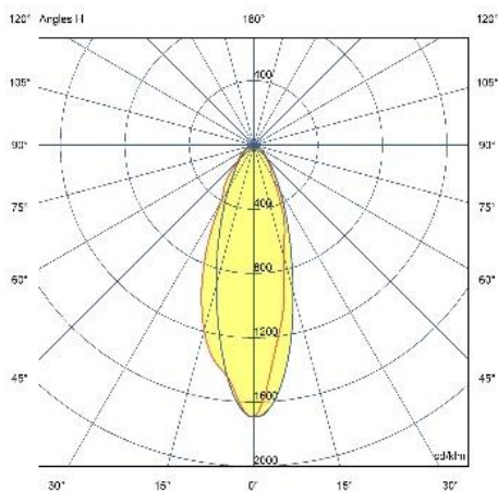
Светлоразпределителна диаграма
