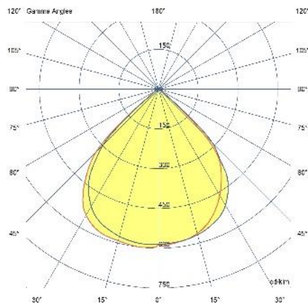
Светлоразпределителна диаграма
