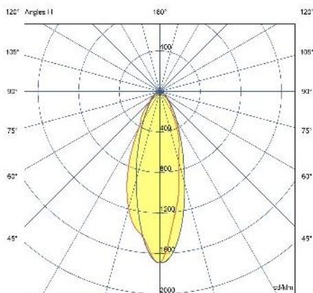
Светлоразпределителна диаграма
