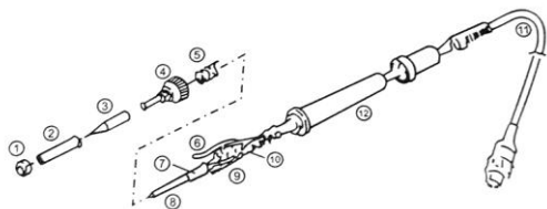
Елементи на поялника
